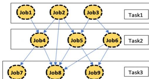
Fig. 2. Job level DAG
