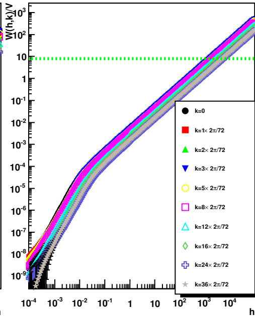
Free energy
